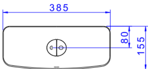
Desenho Técnico
