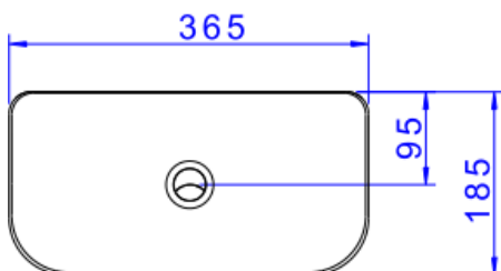
Desenho Técnico
