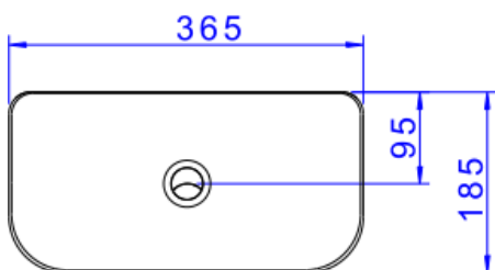
Desenho Técnico
