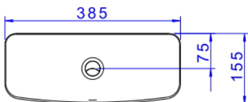
Desenho Técnico
