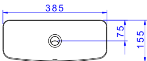
Desenho Técnico
