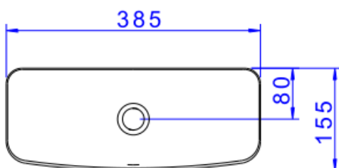
Desenho Técnico
