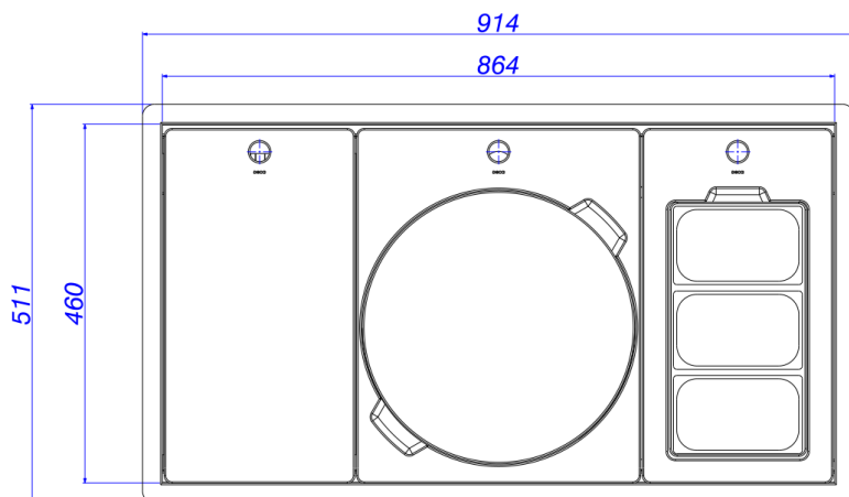
Desenho Técnico
