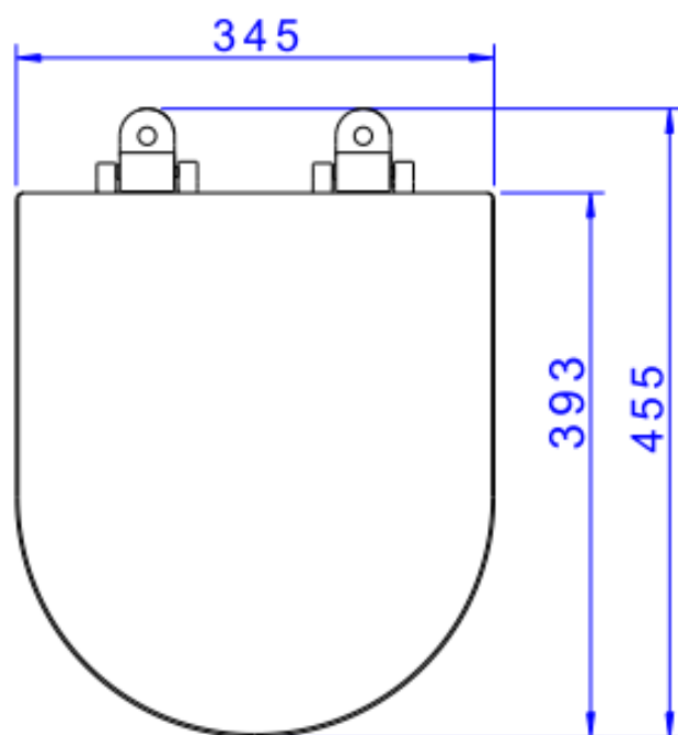
Desenho Técnico
