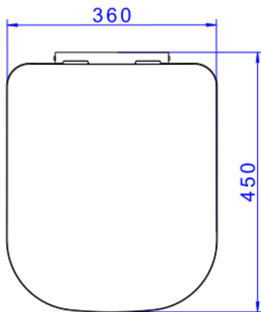
Desenho Técnico
