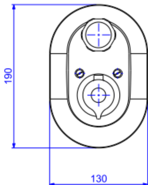
Desenho Técnico
