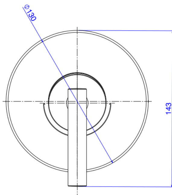
Desenho Técnico
