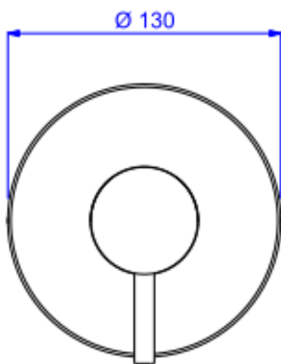
Desenho Técnico
