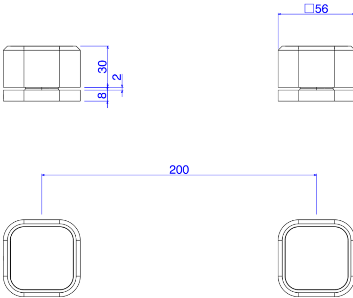
Desenho Técnico
