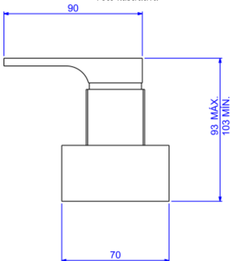
Desenho Técnico
