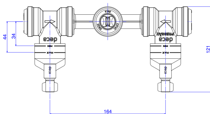
Desenho Técnico
