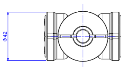
Desenho Técnico
