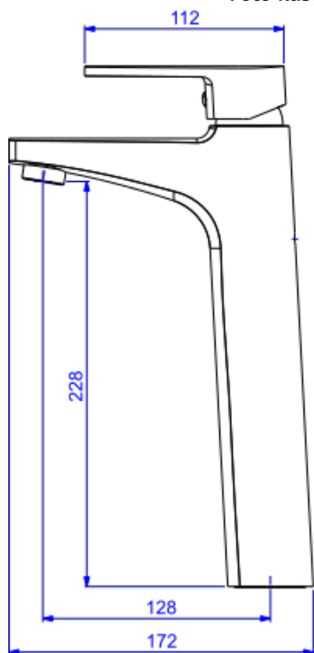
Desenho Técnico
