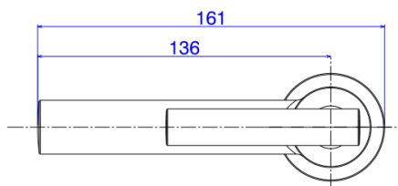
Front view Scale: 1:1
