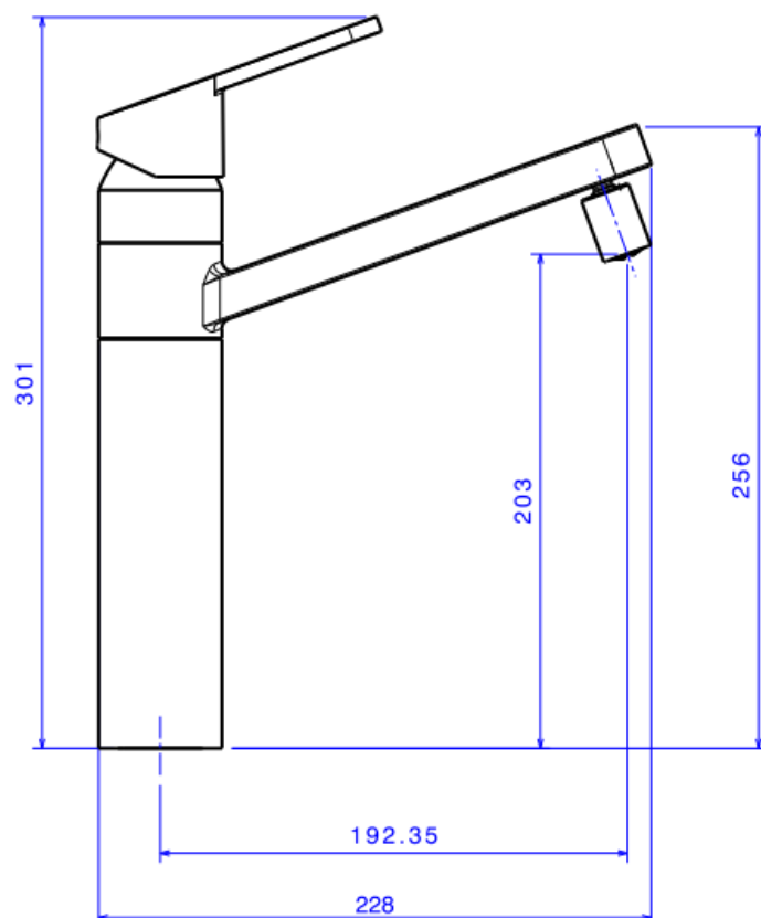
Desenho Técnico
