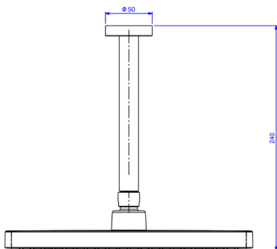
Desenho Técnico
