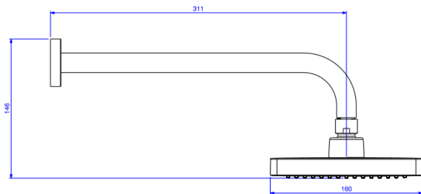
Desenho Técnico
