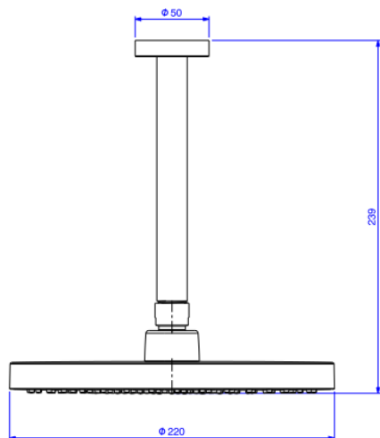
Desenho Técnico
