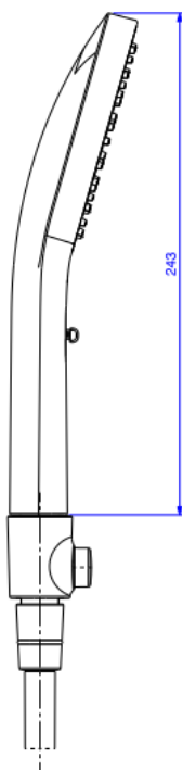
Desenho Técnico
