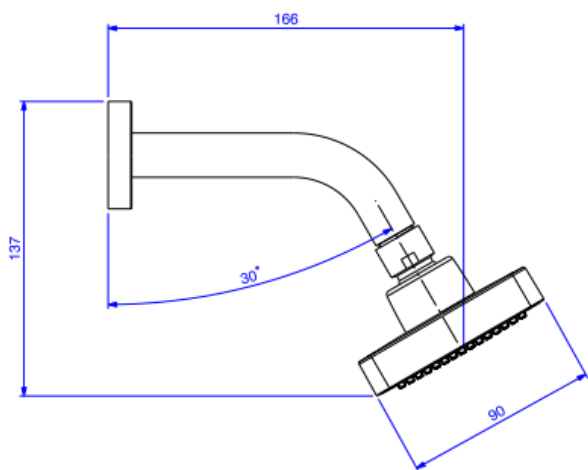
Desenho Técnico
