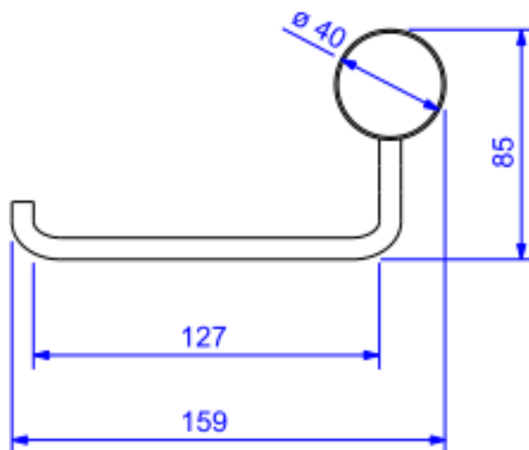
Desenho Técnico
