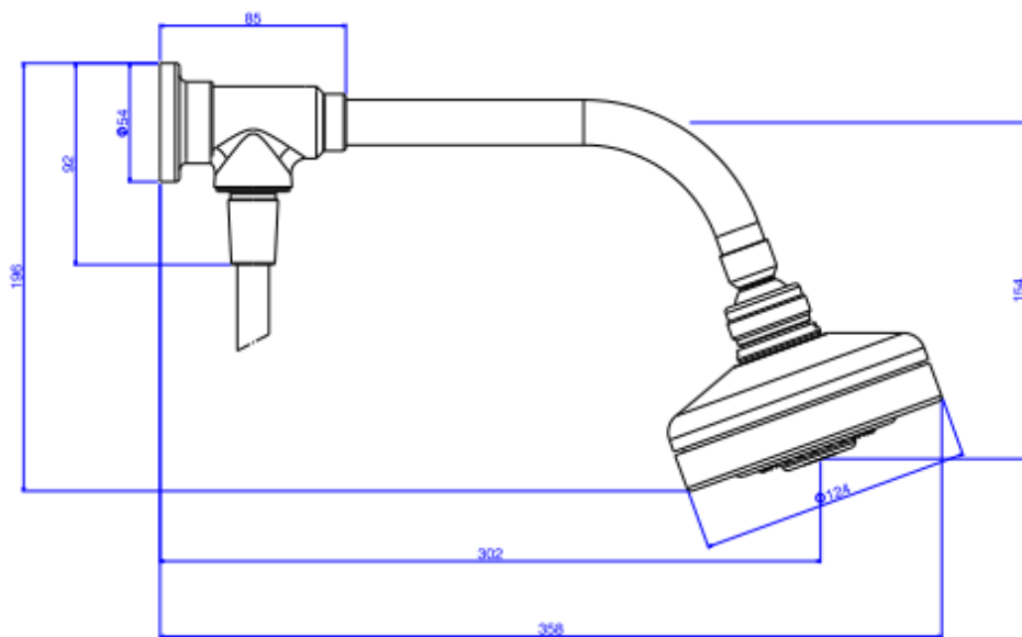
Desenho Técnico
