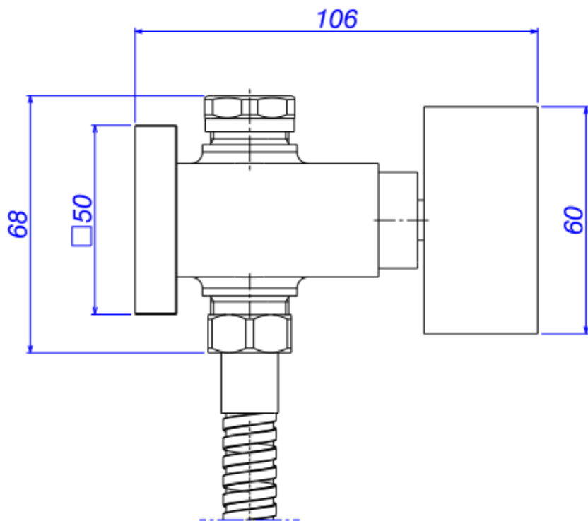
Desenho Técnico
