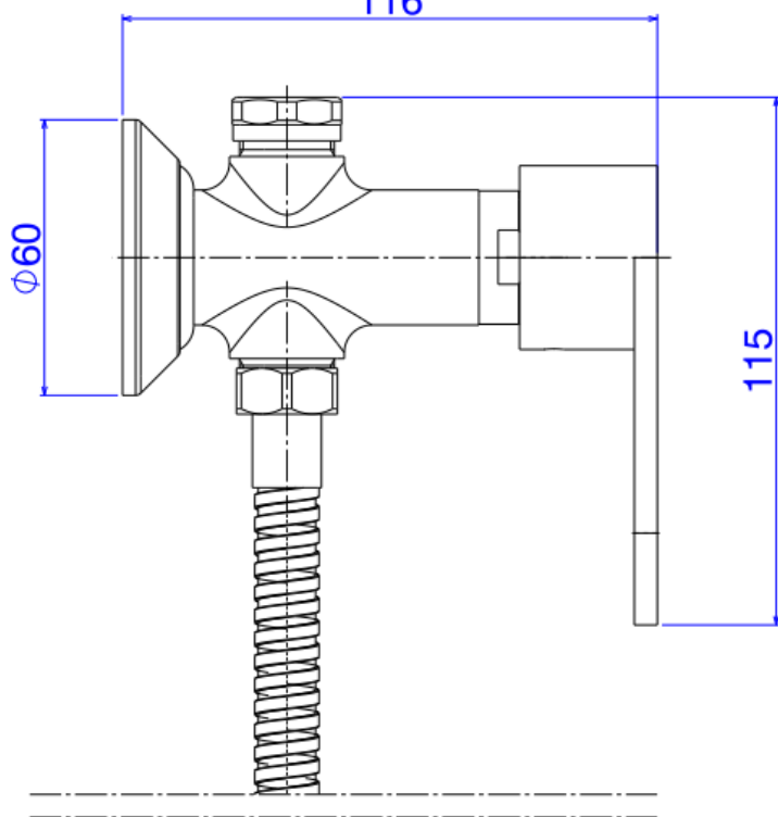
Desenho Técnico
