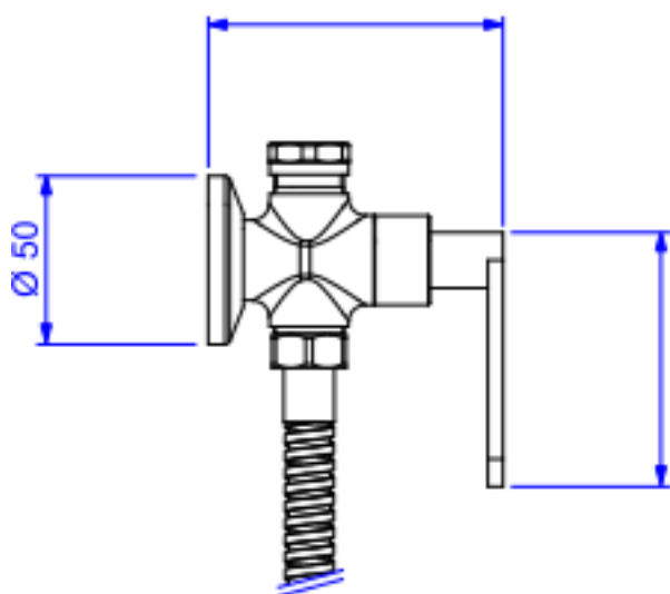
Desenho Técnico
