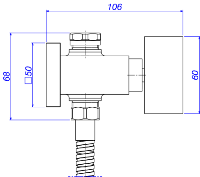
Desenho Técnico
