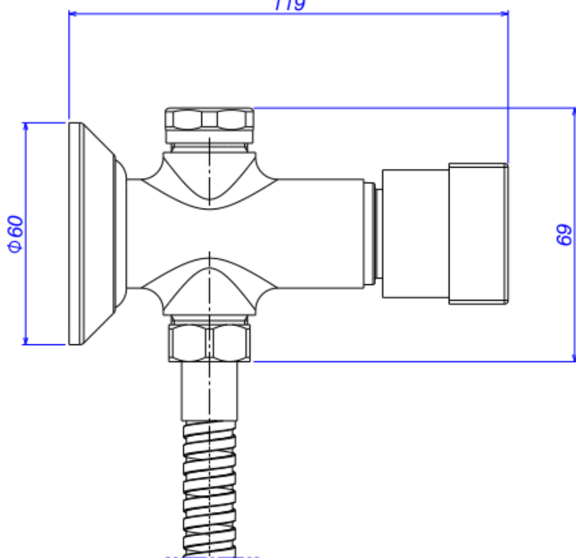
Desenho Técnico
