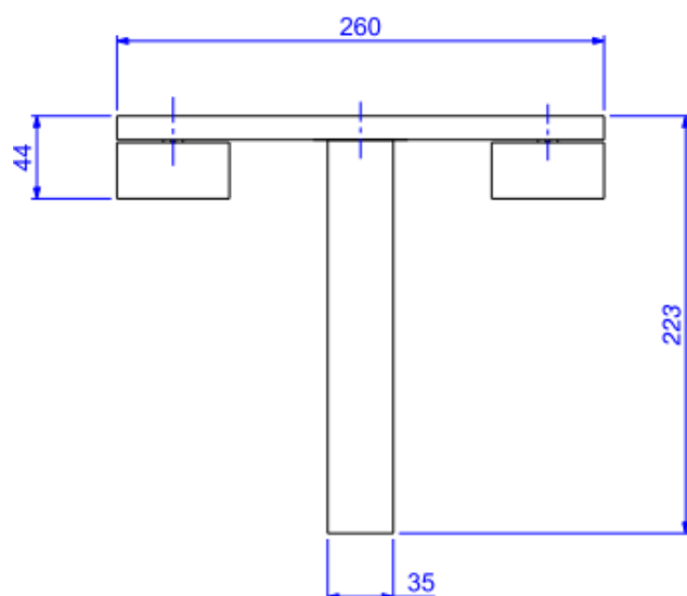
Desenho Técnico
