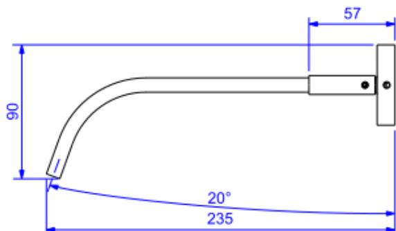
Desenho Técnico
