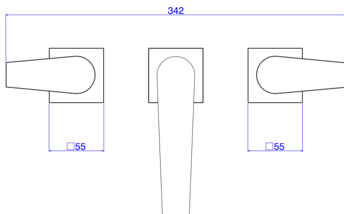
Desenho Técnico
