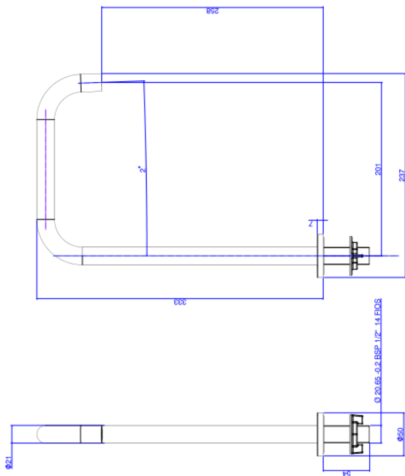
Desenho Técnico
