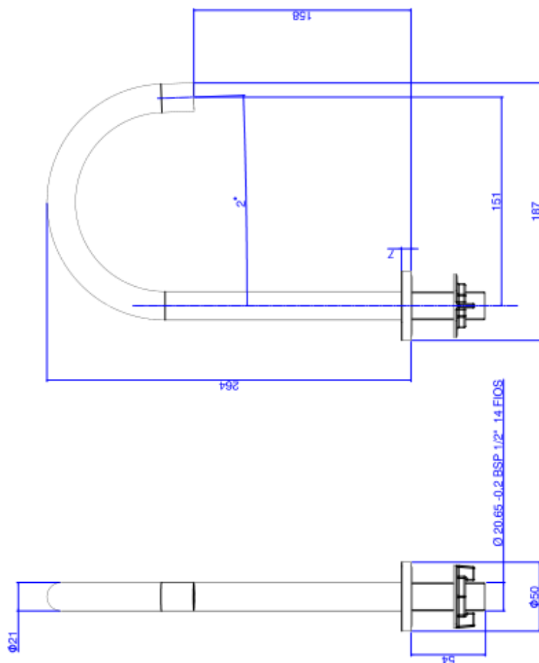
Desenho Técnico
