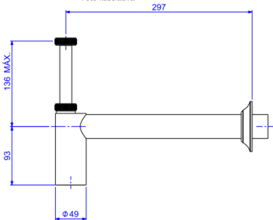
Desenho Técnico
