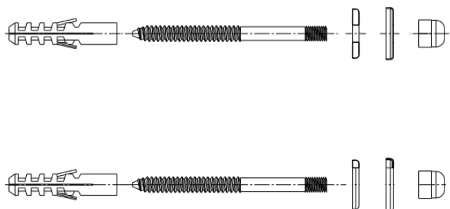
Desenho Técnico
