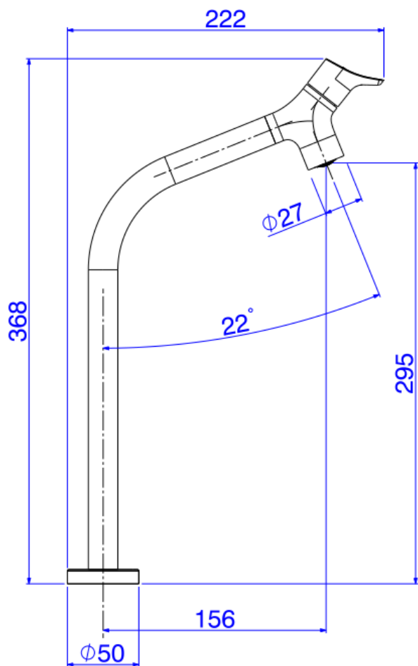
Desenho Técnico
