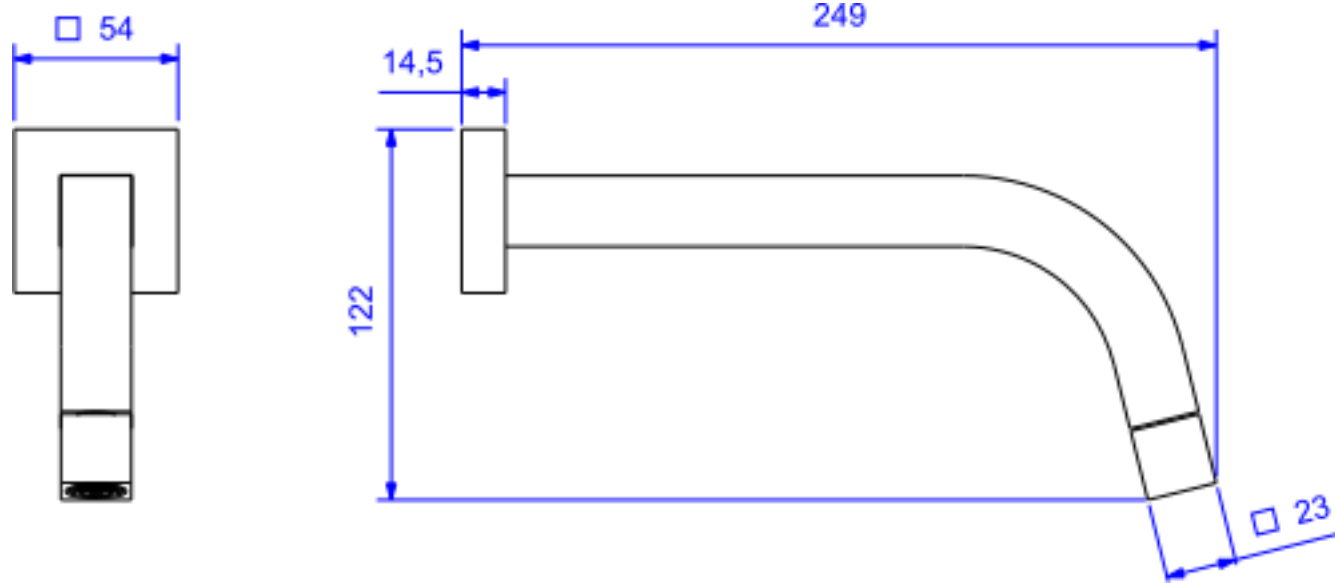
Desenho Técnico
