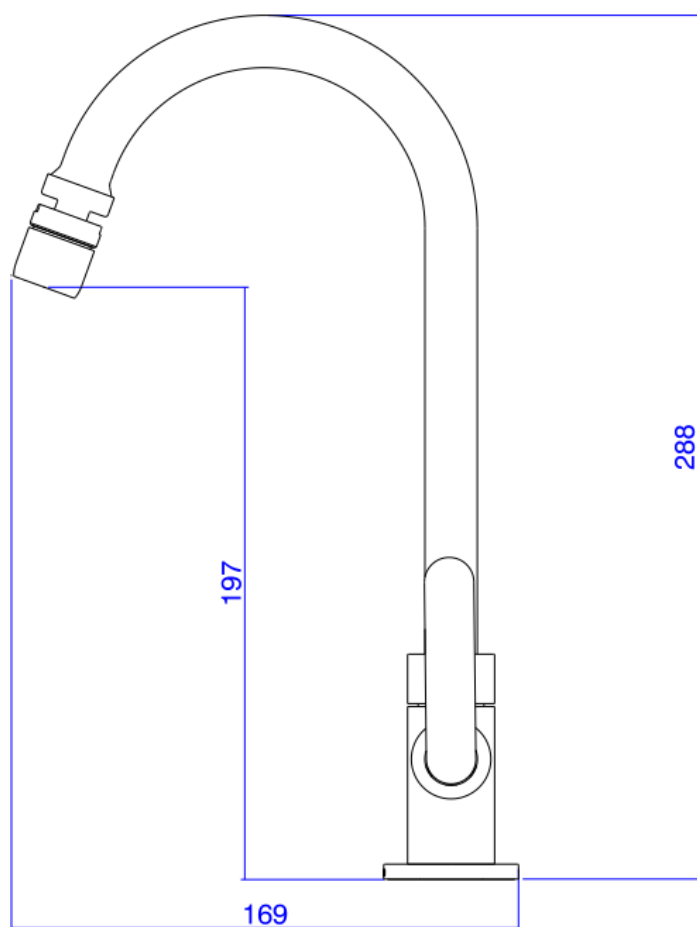
Desenho Técnico
