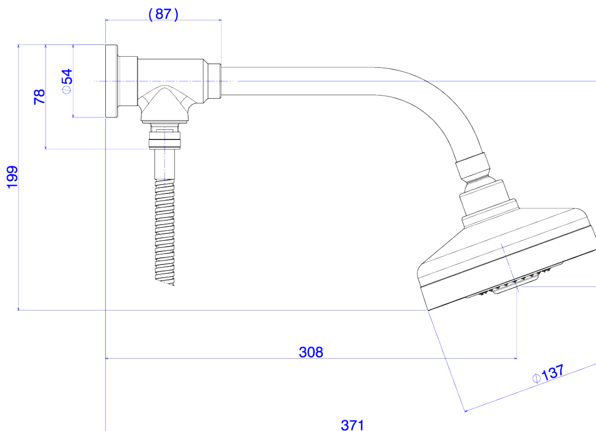
Desenho Técnico
