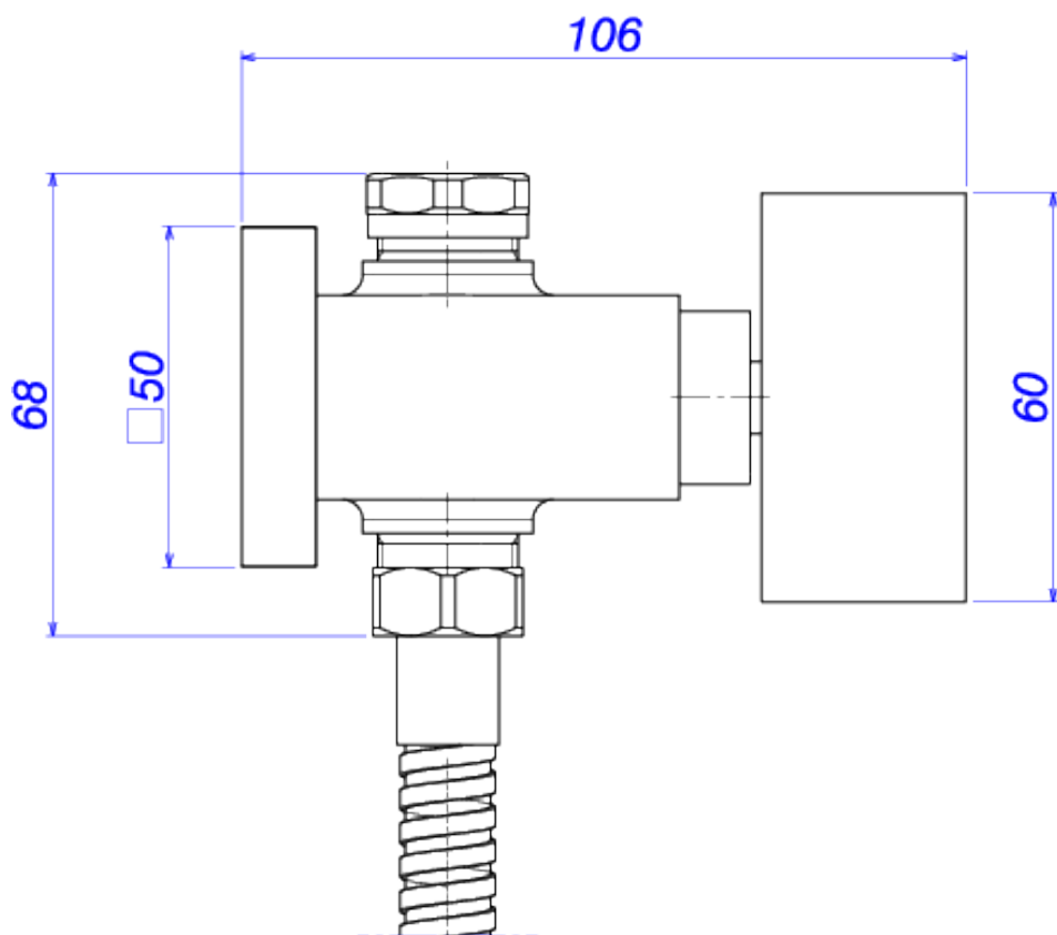
Desenho Técnico
