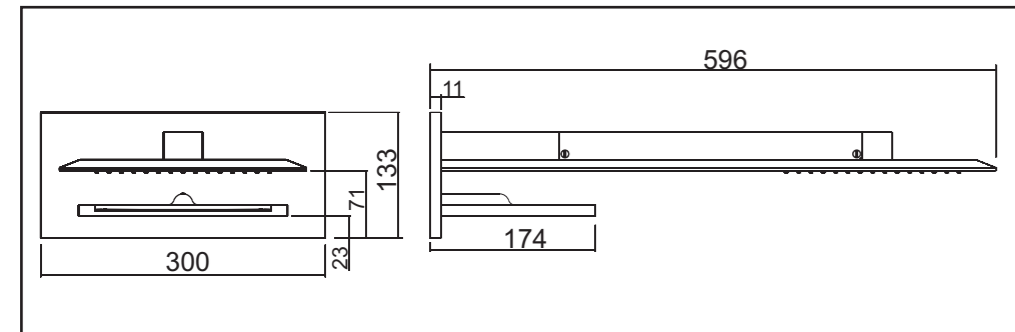
CHUVEIRO TWIN SPA 1978.C.CT.TWN MEDIDAS EM MILIMETROS
