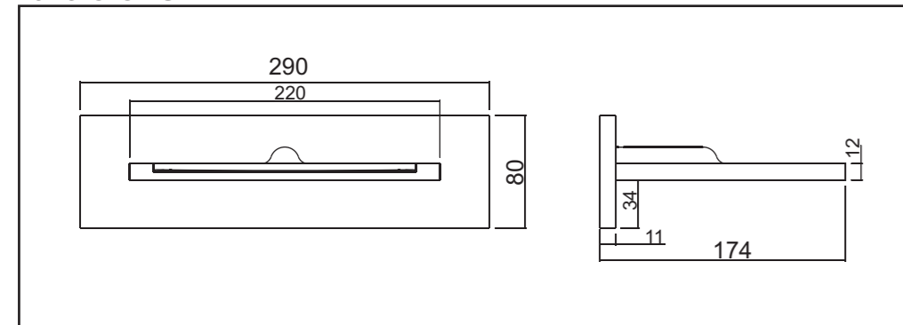
CHUVEIRO CASCATA 1978.C.CAS.TWN
