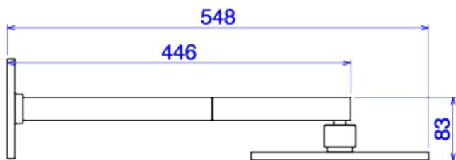
Desenho Técnico
