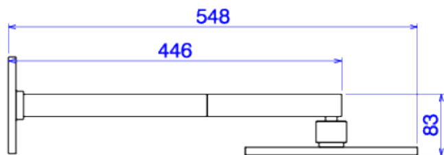
Desenho Técnico
