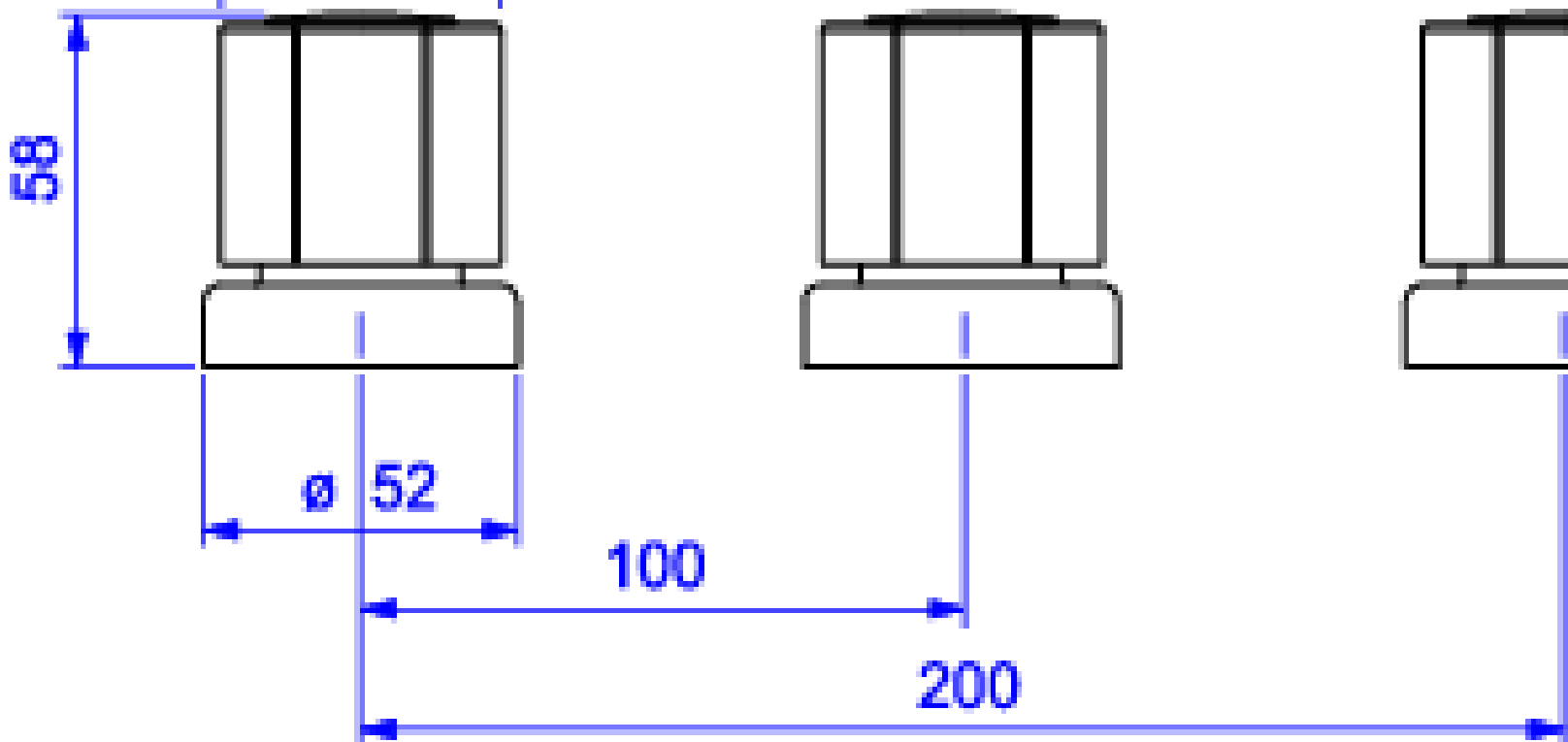
Desenho Técnico
