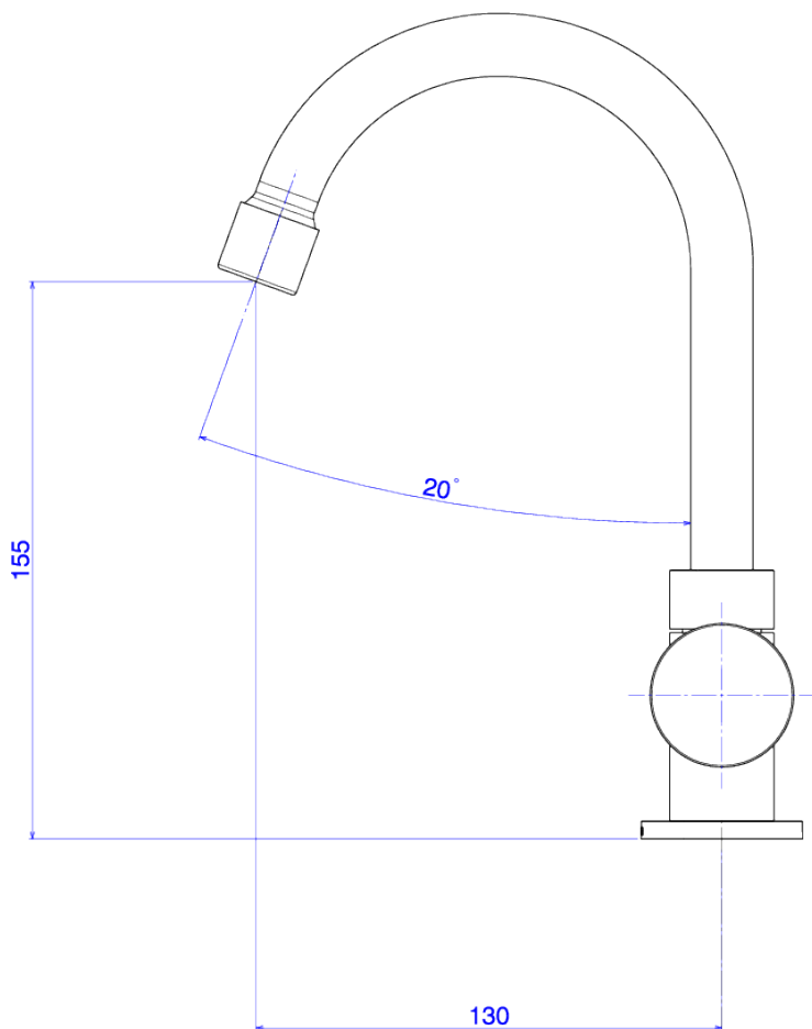
Desenho Técnico
